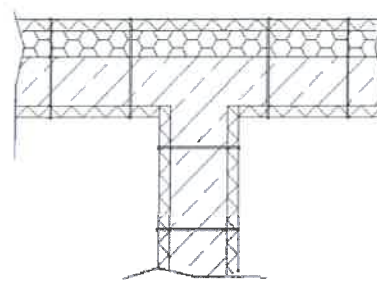
Grundriss: Einbindung Innenwand
