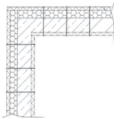
Grundriss: Eckausbildung
