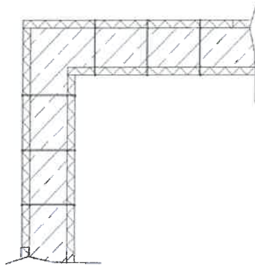
Grundriss: Eckausbildung
