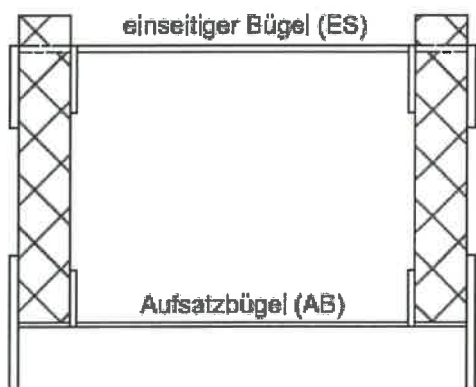
Mauerrost ungedämmt
