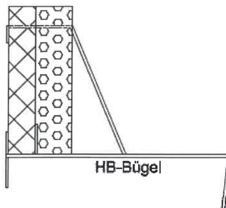
Deckenrost gedämmt
