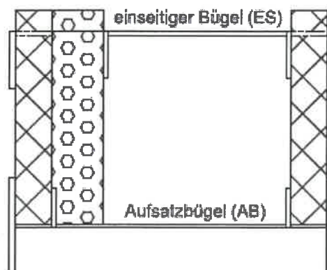
Mauerrost gedämmt
